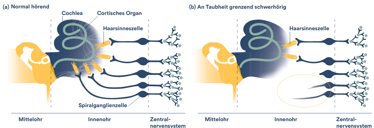
Abb. 4 Schema der Innervierung einer hörgesunden Cochlea (a) und einer Cochlea mit dem für CI-Träger typischen (funktionellen) Verlust der Haarsinneszellen (b) (nach Wilson, Dorman 2008).
